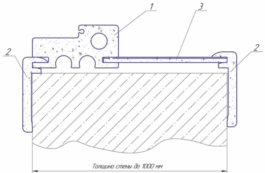
1 - Дверная коробка 80 2 - F наличник 3 - Плоский доборный элемент
