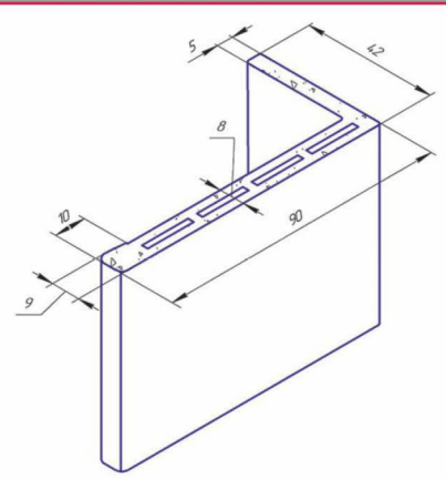
Добор телескопический L184
